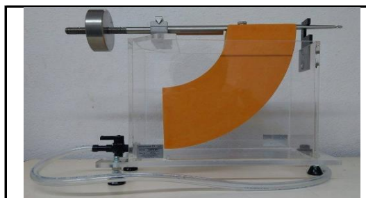
2. F1-12 Equipo de presión hidrostática.
