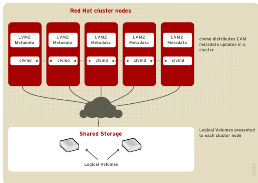
Figura 1.2. Visión general de CLVM
