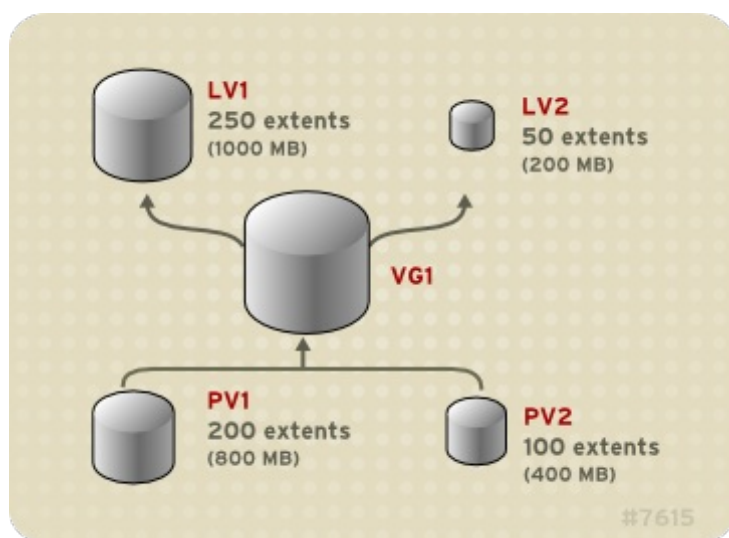
Figura 2.4. Volúmenes lógicos múltiples
