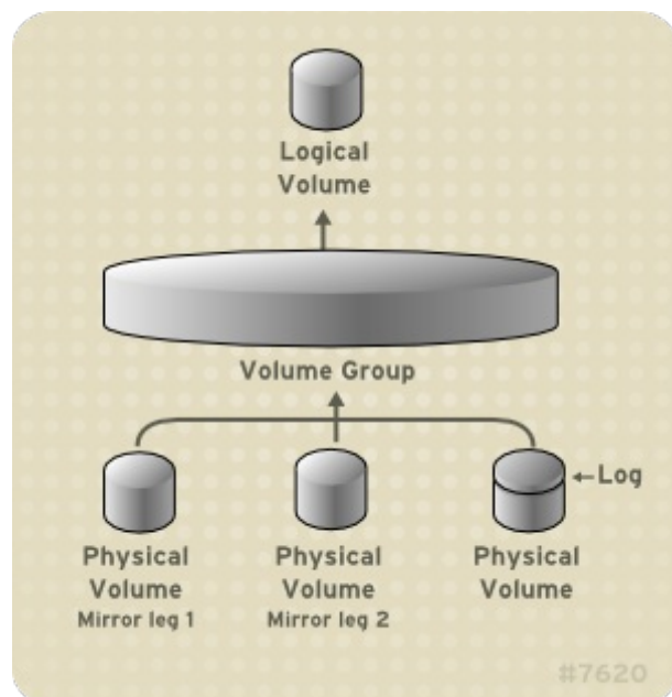
Figura 2.6. Volumen lógico en espejo
