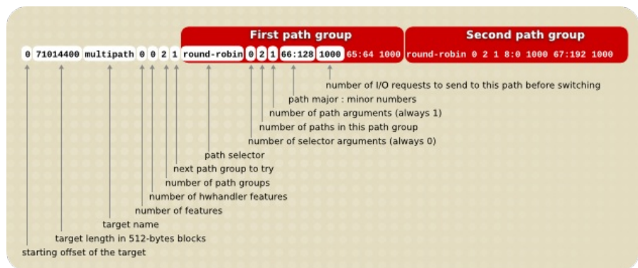
Figura A.1. Destino de mapas multirutas
