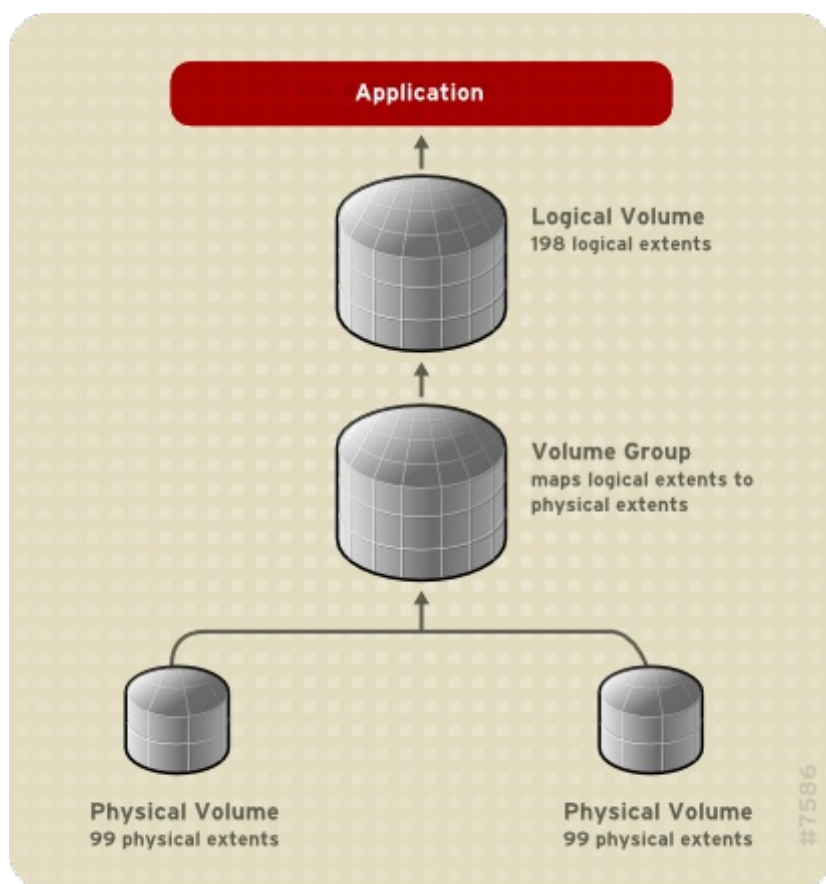
Figura 2.2. Mapas de extensiones
