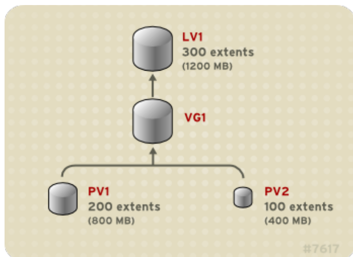
Figura 2.3. Volumen lineal con volúmenes físicos dispares
