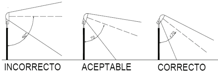
Figura 575.7.e) ángulos de inclinación de proyectores
