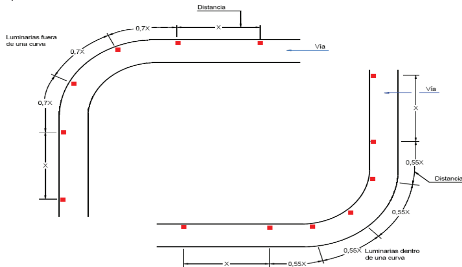
Figura 510.5.2 a. Disposición de luminarias en trayectos curvos
