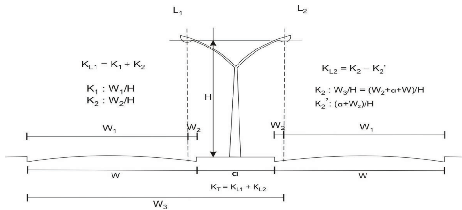
Figura 530.2.2 h. Localización central doble
