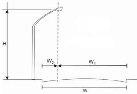
Figura 530.2.2 a. Determinación del Coeficiente de Utilización
