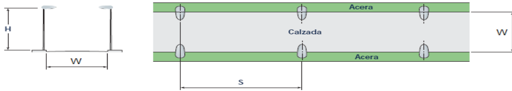
Figura 510.5.1 d. Disposición Bilateral opuesta
