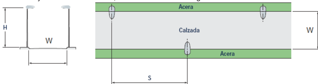
Figura 510.5.1 c. Disposición Bilateral alternada
