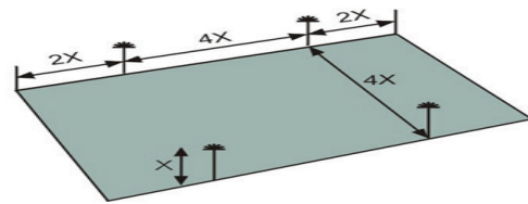
Figura 560.1 b. Ubicación de mástiles laterales al área
