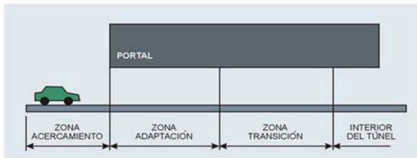
Figura 570 Zonas lumínicas de un túnel
