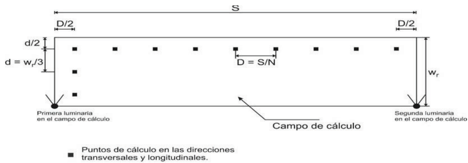
Figura 530.3.1. Puntos de cálculo para la iluminación
