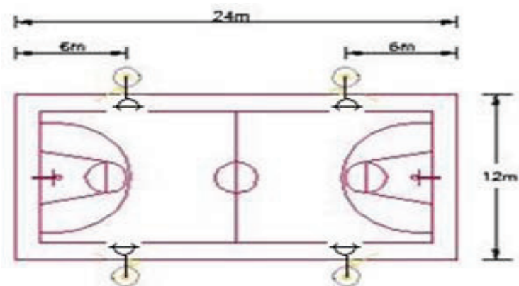
Figura 560.3.3 b. Cancha múltiple sencilla
