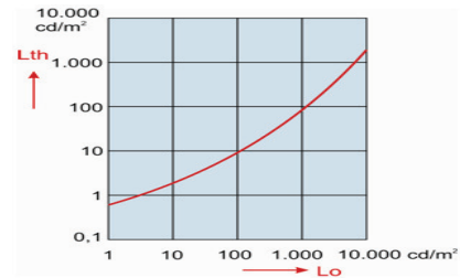
Figura 570.3 a. Nivel de iluminancia en túneles
