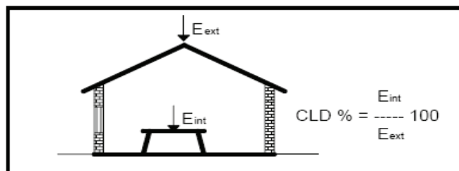
Figura 410.2.1 El coeficiente de luz diurna
