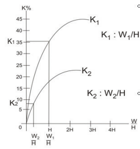
Figura 530.2.2 b. Curvas de coeficiente de Utilización
