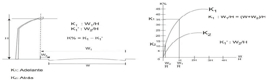
Figura 530.2.2 e. Luminaria sobre la acera
