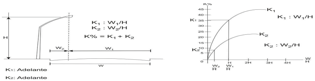
Figura 530.2.2 d. Luminaria sobre la calzada
