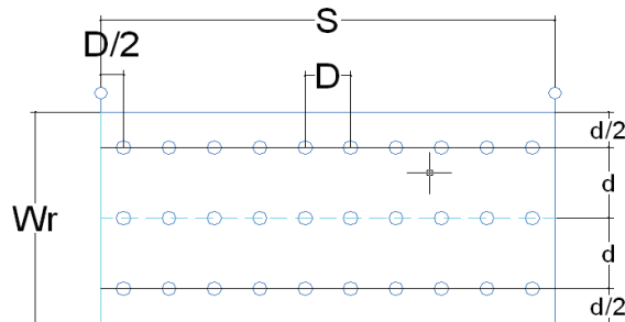
Figura 540.2.2. Malla de medición para iluminancia y luminancia
