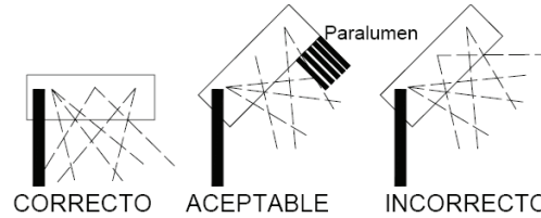
Figura 575.7.a) Control del flujo luminoso de proyectores
