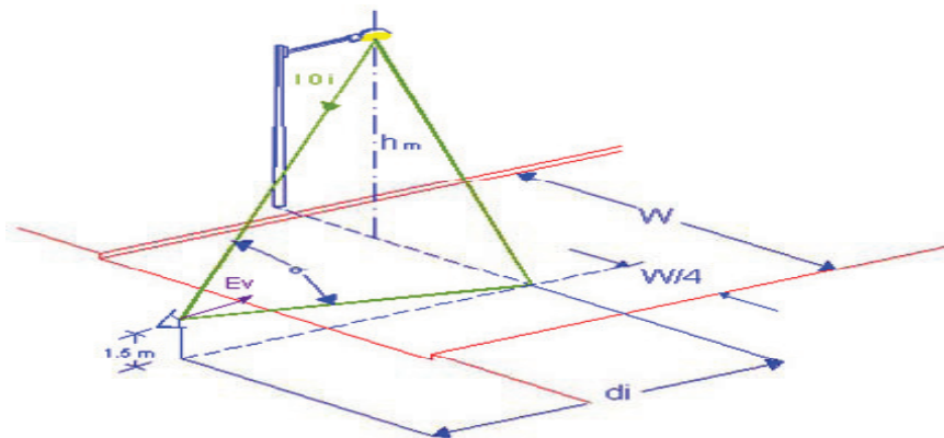
Figura 530.4.6 Cálculo de Luminancia de Velo
