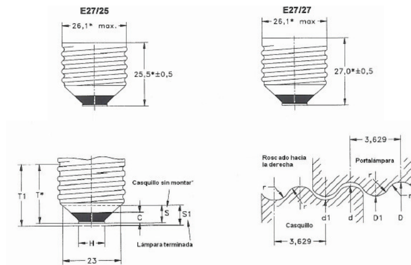
Figura 310.1.1 Dimensiones del casquillo de una bombilla en milímetros.
