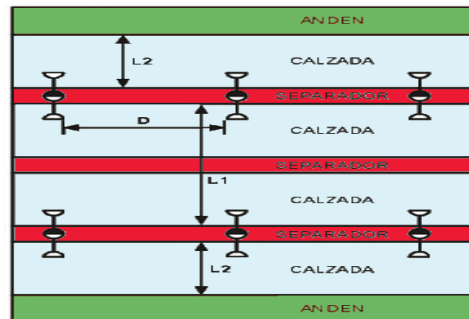
Figura 510.5.1 f. Disposición Doble central doble
