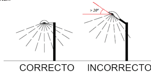
Figura 575.7.b) Ángulos de inclinación de las luminarias
