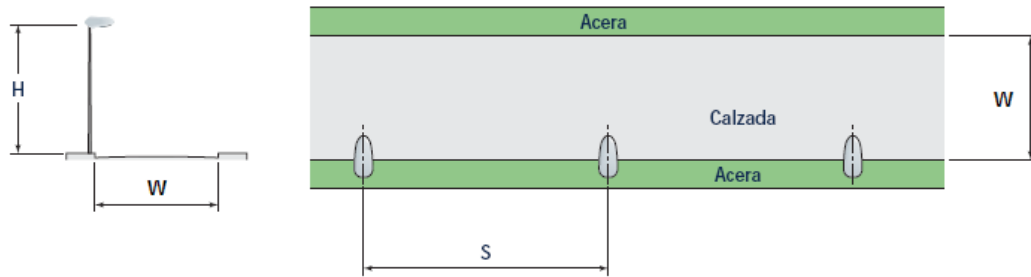
Figura 510.5.1 a. Disposición Unilateral
