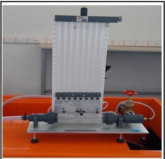
2. F1-15 Demostración teorema de Bernoulli
