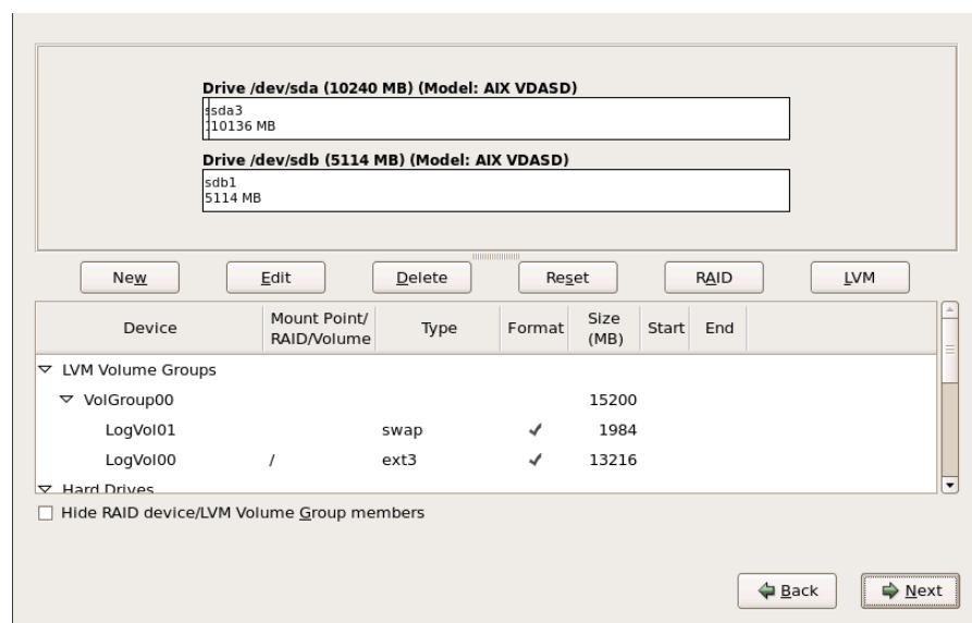
Figura 16.38. Particionamiento en IBM System p
