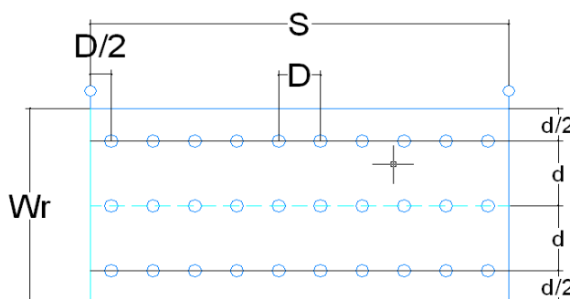
Figura 540.2.2. Malla de medición para iluminancia y luminancia
