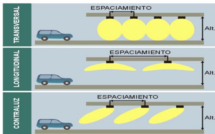
Figura 570.6. Tipos de luminarias para túneles, según su distribución luminosa
